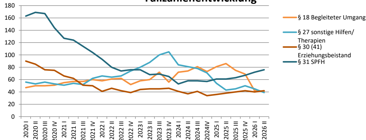
Fallzahlenentwicklung
